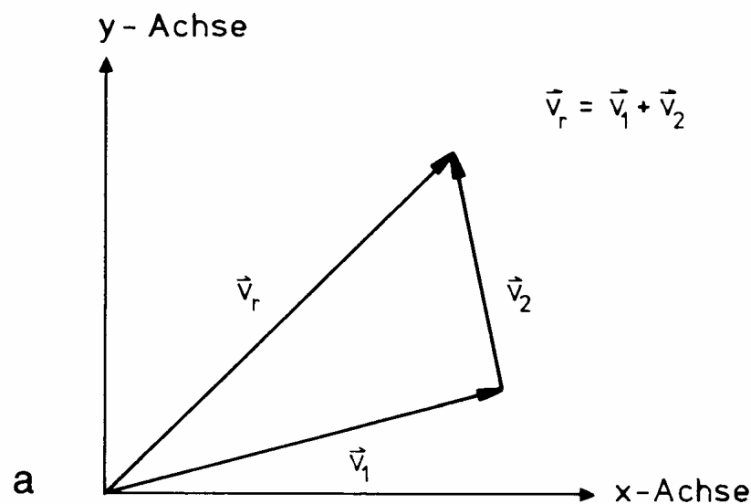
Addition (a) und Subtraktion (b) von Vektoren.
