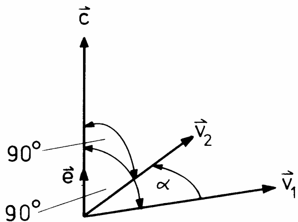
Zum Vektorprodukt von Vektoren
